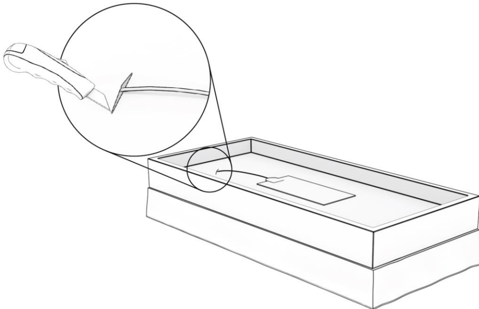
Figuur 3: Positionering van het verwarmingselement en doorvoersleuven snijden in de schuimkern en onderkant van de tijk.
